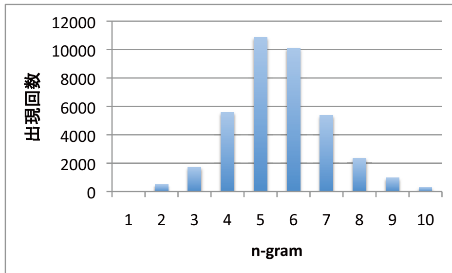
図4 n -gram 長の分布
