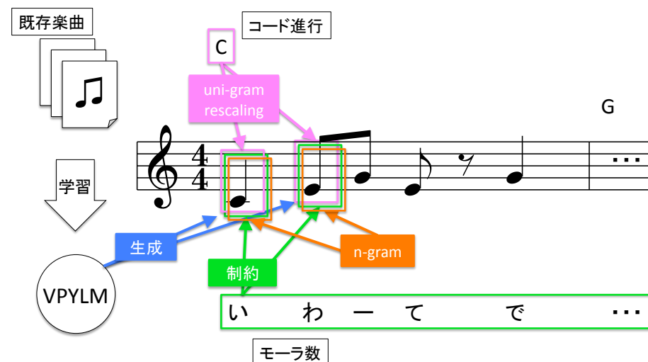
図 1 提案手法の概要図
